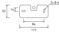
SCHÉMA DE FIXATION FIXING DETAILS
